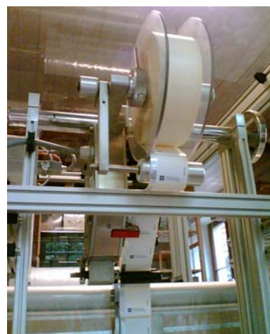
Integrierter Etikettenspender
